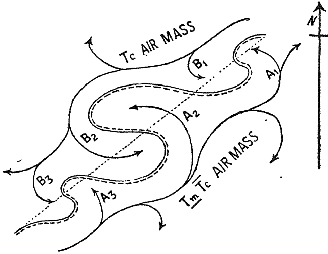
चित्र ५९—Tc और TmTc वायु राशियों के बीच अग्रभाग का बनना। विन्दी रेखा विक्षोभ के पहले अलगाव दर्शाती है।
